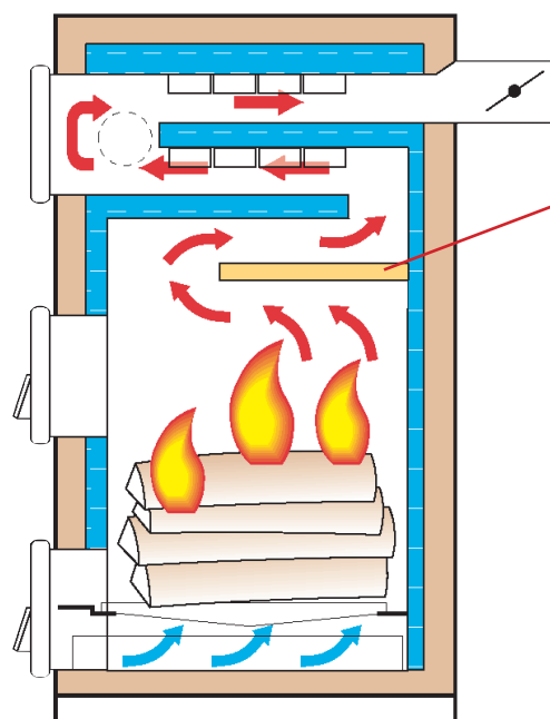
PUUOSAN POIKKILEIKKAUS
